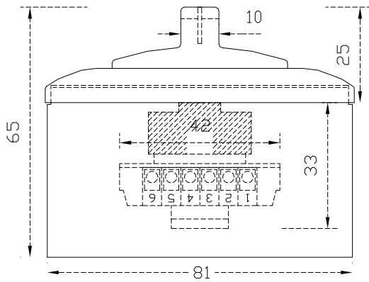
LSPR IN ENKELVOUDIGE OPBOUWDOOS AP1
