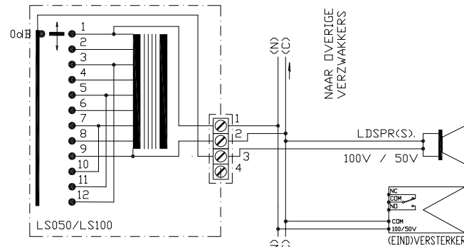
SCHAKELVOORBEELD ZONDER OVERBRUGGING VAN DE VERZWAKKER BIJ OPRDEP
