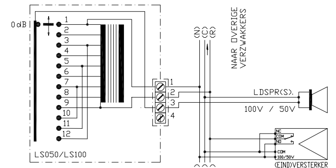
SCHAKELVOORBEELD MET VERPLICHTE, ONVERZWAKTE OPRDEP
